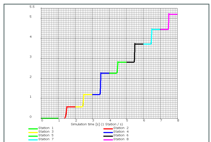
Längsdehnungen in den jeweiligen Umformstationen
