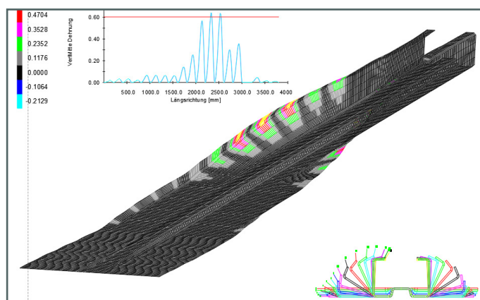
Abb. 2: COPRA® RF zeigt Werte und Positionen der Längsdehnungen an
